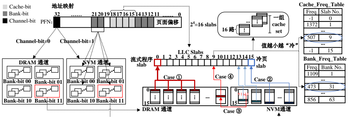
Fig. 12 Hybrid Memory Management Framework 图 12 混合内存管理在整个内存体系上的应用架构
